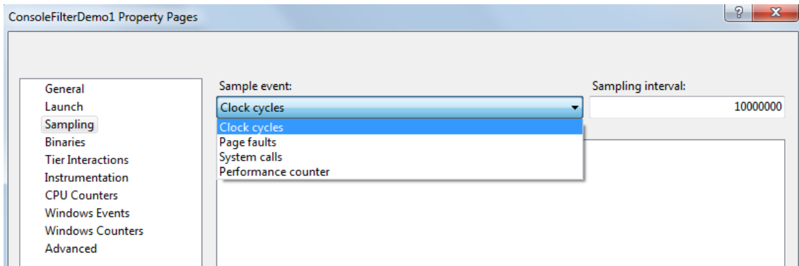
5. ábra. Mintavételező profiling munkamenet (sampling) tulajdonságai.
