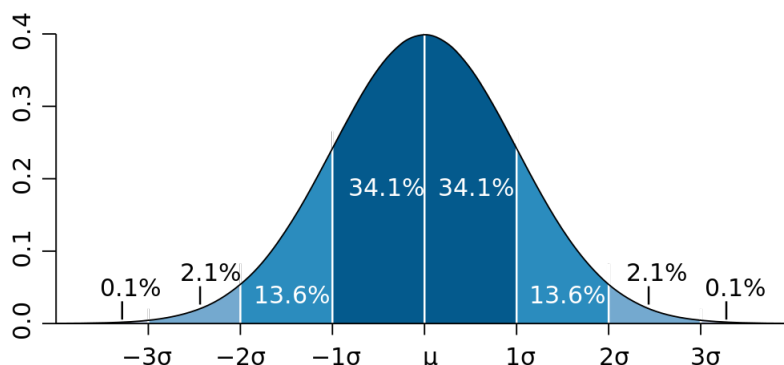
1. ábra. Konfidenciaintervallumok
