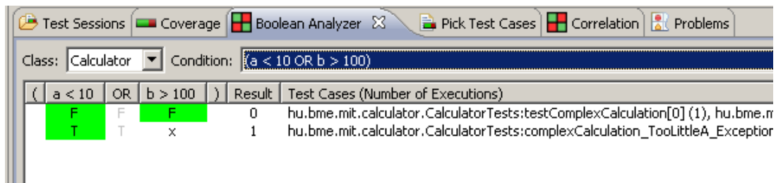
5. ábra: Feltétel lefedettség vizsgálata
