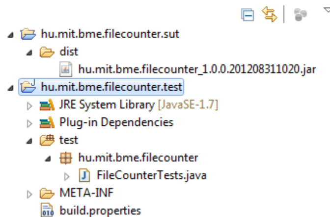
8. ábra: FileCounter teszt projekt vázlata
