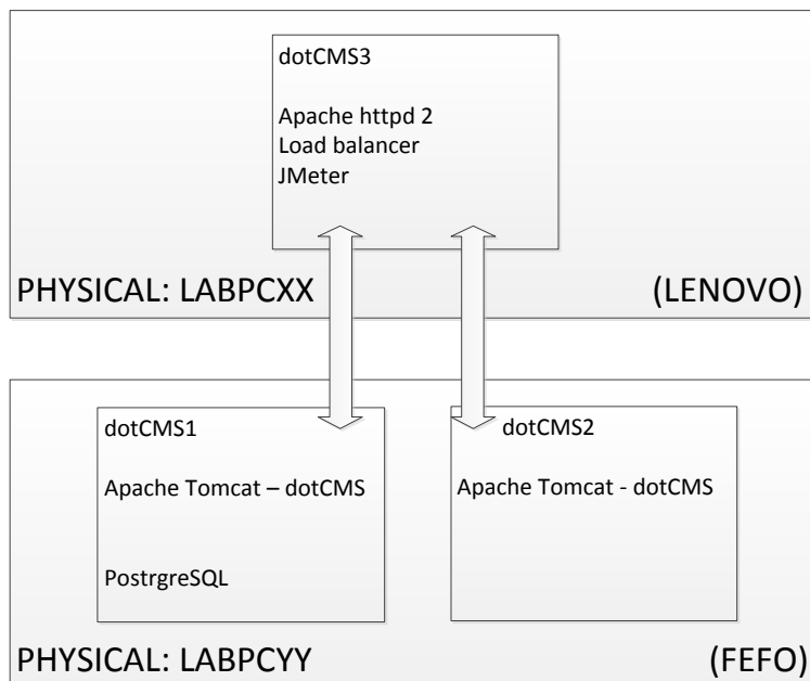
Ábra 1 Mérési elrendezés
