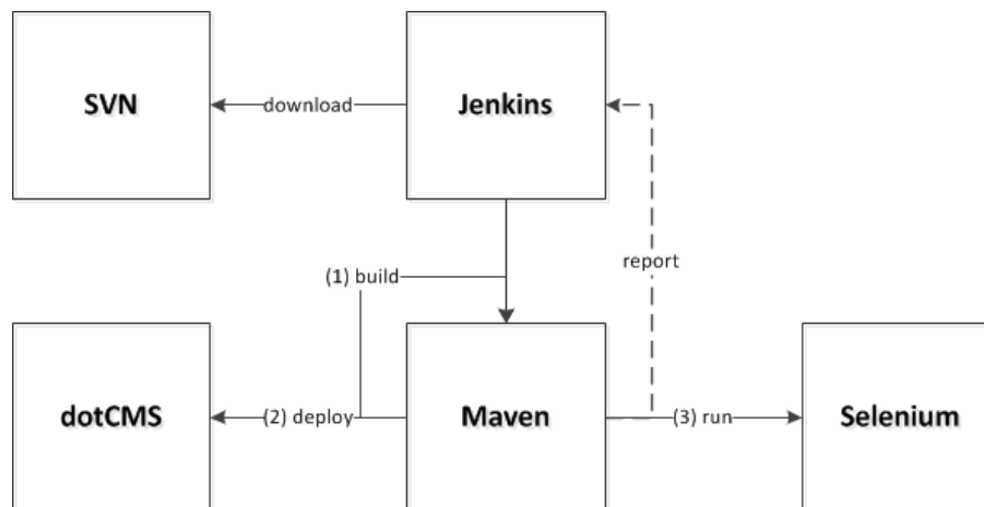
2. ábra. Architektúra ábra
