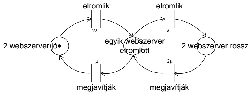
18. ábra: Két webszerver Petri hálós modellje
