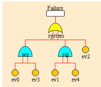
4. ábra: webes rendszer SHARPE hibafája
