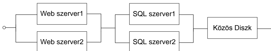
9. ábra: Webes rendszer RBD-je
