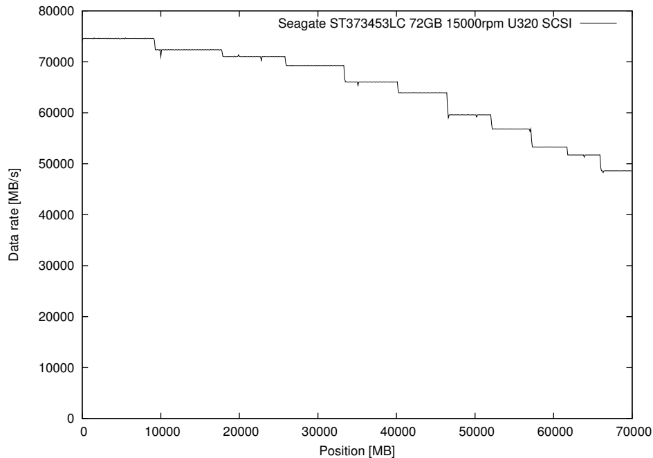
1. ábra. Merevlemez áteresztőképessége olvasási hely függvényében (zónás felépítés)
