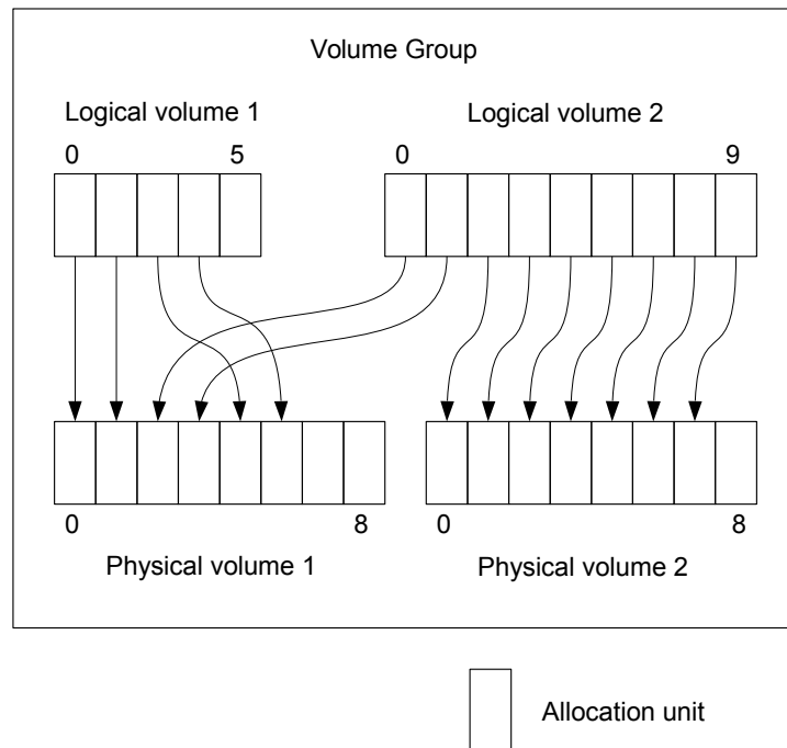
2. ábra. Példa fizikai kötetek allokációs egységeinek hozzárendelés logikai kötethez
