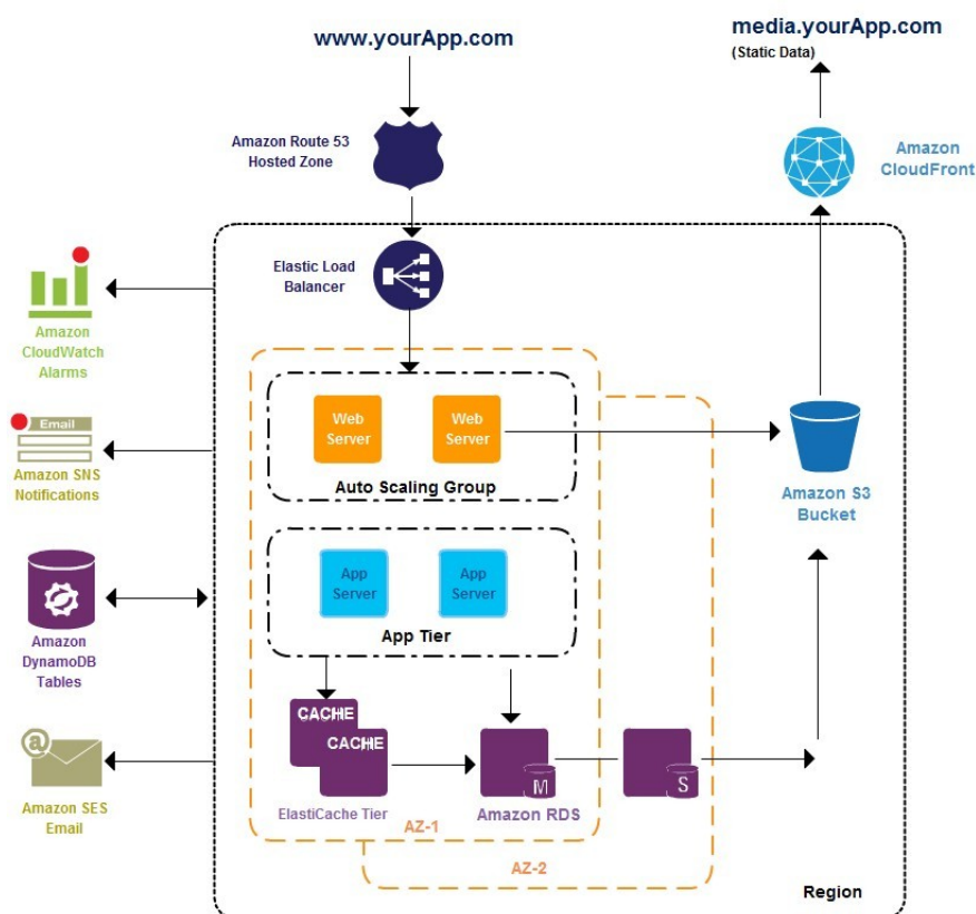
Figure 2: Az AWS szolgáltatásinak felhasználása egy komplex szolgáltatás kialakítására
