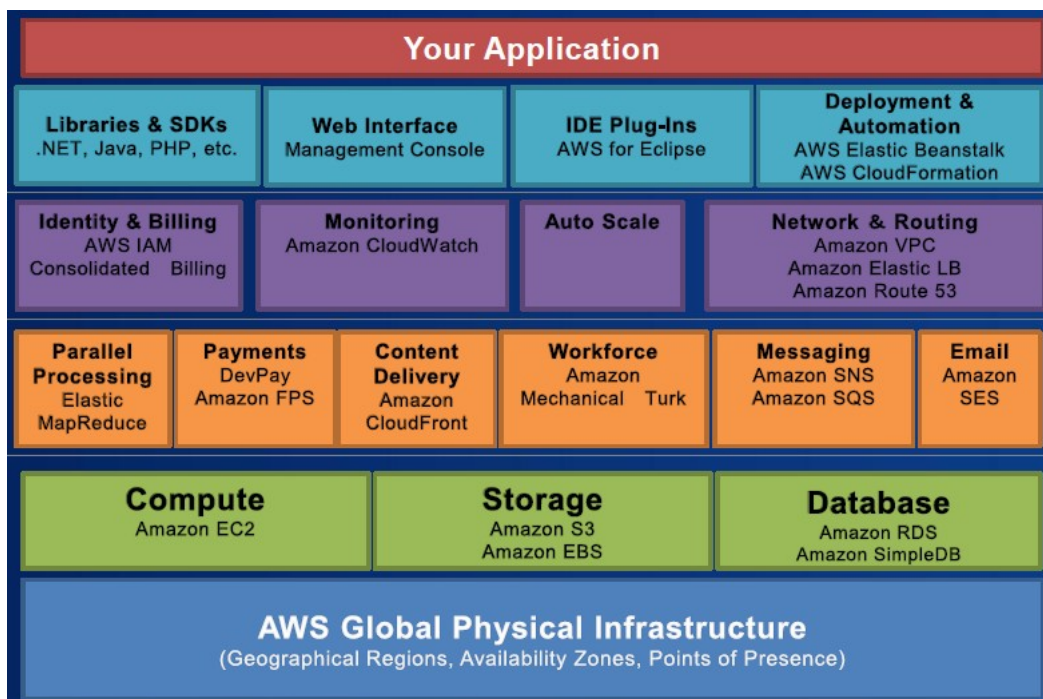
Figure 1: Az AWS szolgáltatások egymásra épülése
