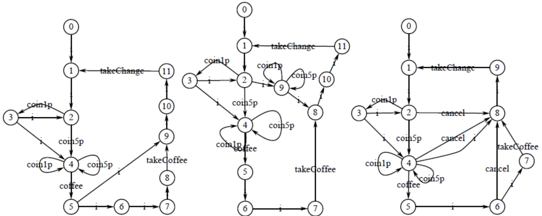
b. LTS 4 : AnticipatingMachine
